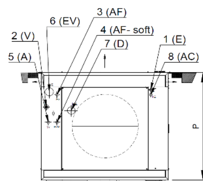
UKŁAD MASZYNY
